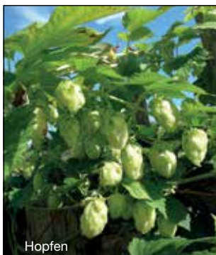
Hopfen
